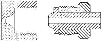
CGA 702 1.125-14NGO-RH-INT
