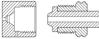
CGA 703 1.125-14NGO-LH-INT
