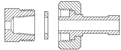
CGA 705 1.125-14UNS-2A-RH-EXT
